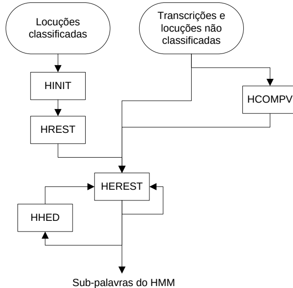
Figura 5.4 Sistema de treinamento da ferramenta HTK.
