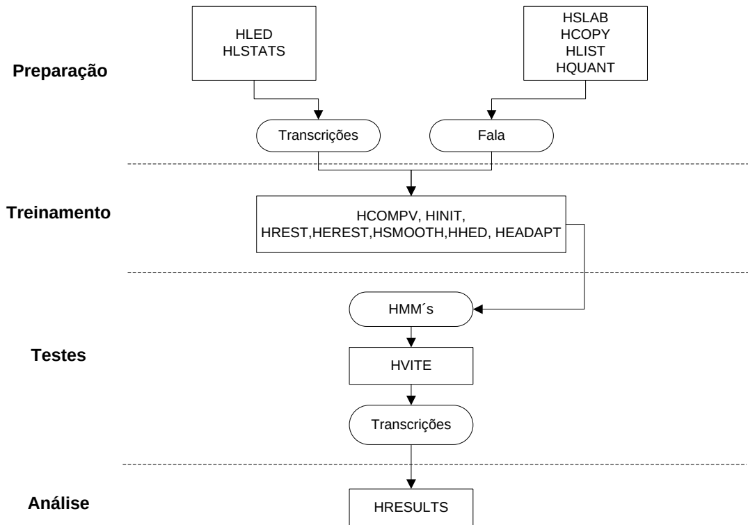
Figura 5.3 Estágios do processamento da ferramenta HTK.
