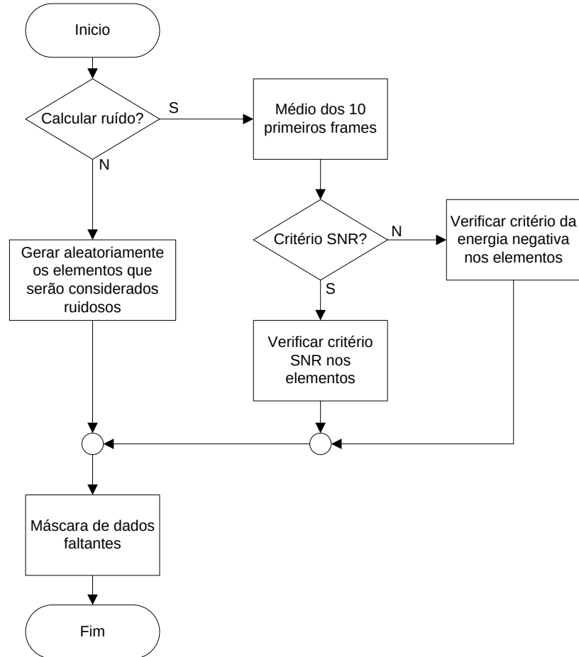
Figura 5.5 Fluxograma da criação da máscara de dados.
