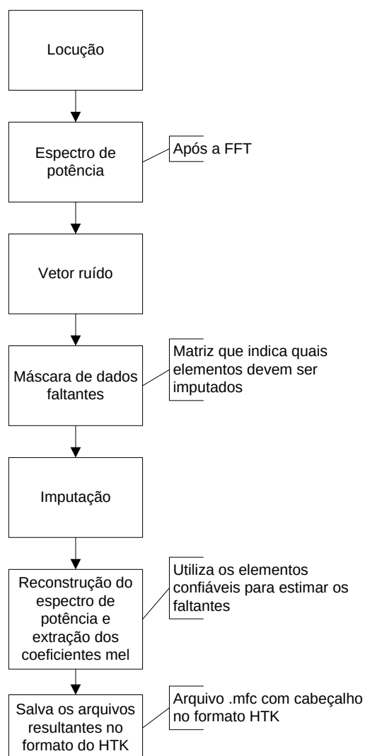
Figura 5.8 Diagrama em blocos da plataforma desenvolvida.
