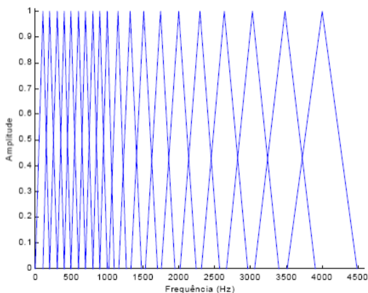
Figura 2.3 Banco de filtros da escala Mel [9].
