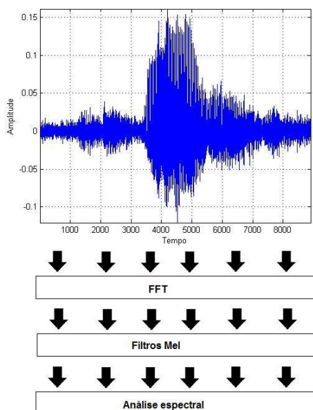
Figura 5.1 Transformando locuções em espectrogramas mel.
