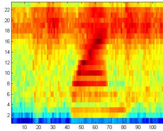
Figura 6.1 Espectrograma de uma locução sem ruído.
