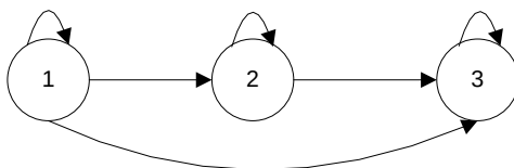
Figura 2.6 Cadeia de Markov esquerda-direita
