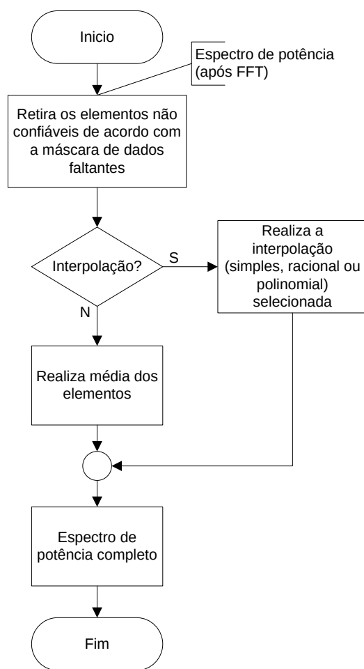
Figura 5.6 Fluxograma da interpolação na reconstrução dos dados.
