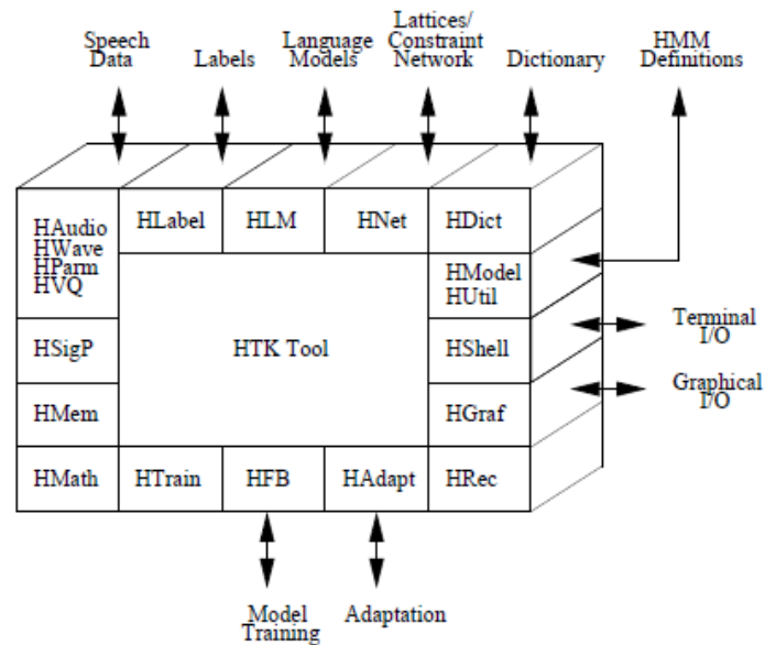
Figura 5.2 Arquitetura da ferramenta HTK [44].
