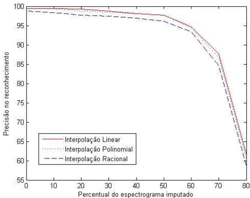
Figura 6.4 Resultados das interpolações propostas.
