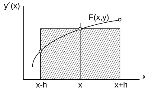
Figura 4.2 Integração Numérica.
