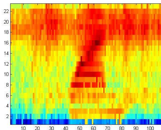
Figura 6.3 Espectrograma reconstruído.
