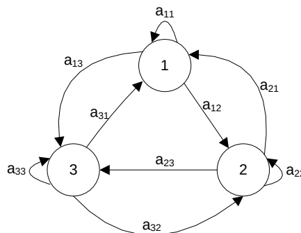
Figura 2.5 Cadeia de Markov de 3 estados.
