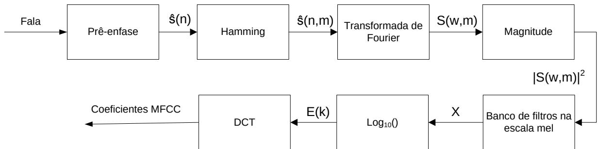
Figura 2.4 Extração dos coeficientes MFCC [14].
