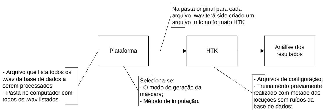
Figura 5.7 Diagrama em blocos do sistema.
